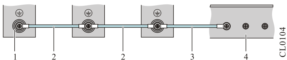
Рисунок в приложении Е-1 Экипотенциальная связь устройства
