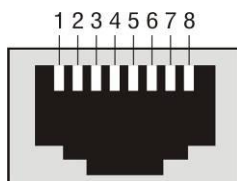
Рисунок в приложении Г-2 Патрон RJ45
