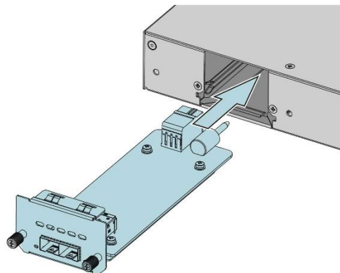
Рисунок В-8 Установите интерфейсную карту
