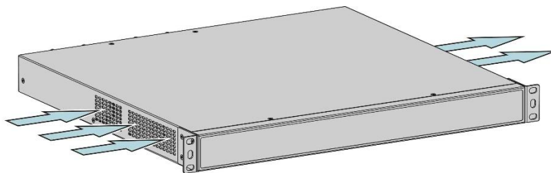
Рисунок А-5 Воздушные проходы серии S3230
