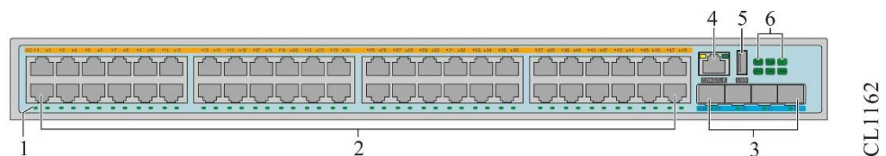
Рисунок А-3 Схема передней панели S3230-54TXP-AC(V1)
