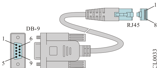
Рисунок в приложении Г-1 Кабель консоли
