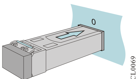
Рисунок Г-13 Установите модуль SFP
