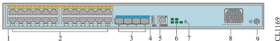
Рисунок А-2 Схема передней панели S3230-28TXP-AC(V1)
